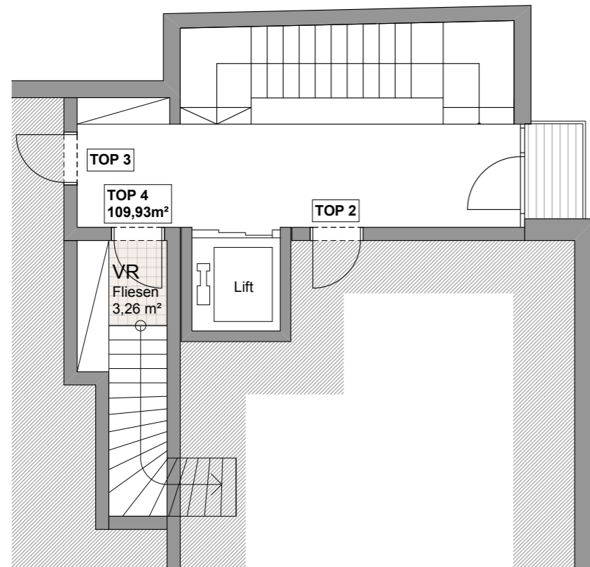
Eingangssituation 2. Obergeschoß
